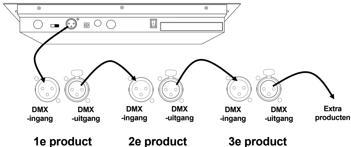
DMX-kabeldiagram
